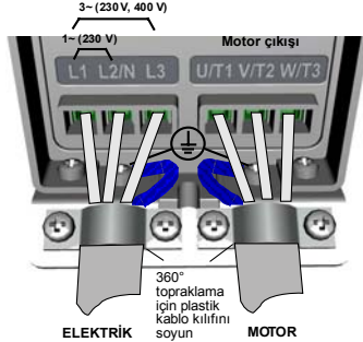
Şekil 7: Vacon 20 elektrik bağlantıları, MI1
