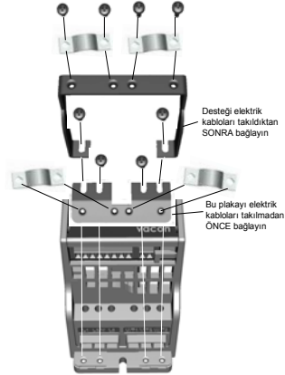
Şekil 5: PE'nin (plaka ve API kablo desteği) bağlanması, MI1 - MI3
